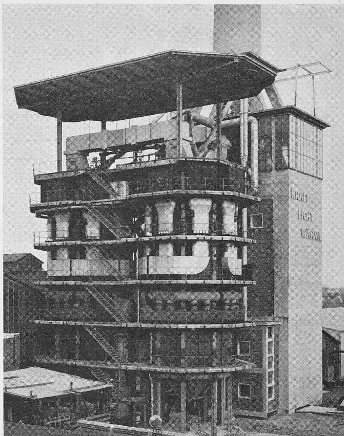
Bild 24. Die Gasturbinenanlage Oberhausen von 13 MW. Vorn der kohlenstaubeu- gefeuerte Lufterhitzer, hinten das Maschinenhaus
