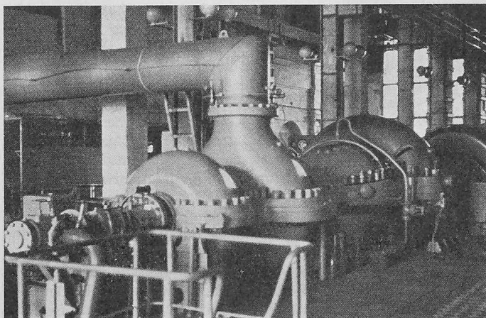
Bild 23. Maschinengruppe der Anlage Nowokaschirsk
