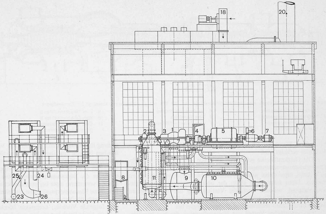
Bild 7. Kombinierte Anlage mit Gasturbine von 10 000 kW und Flash-Verdampfer zur Erzeugung von 63 t/h Süsswasser. Die indirekte Heizung im Luftheritzer gestattet die Verwendung von verschiedenartigen Brennstoffen
