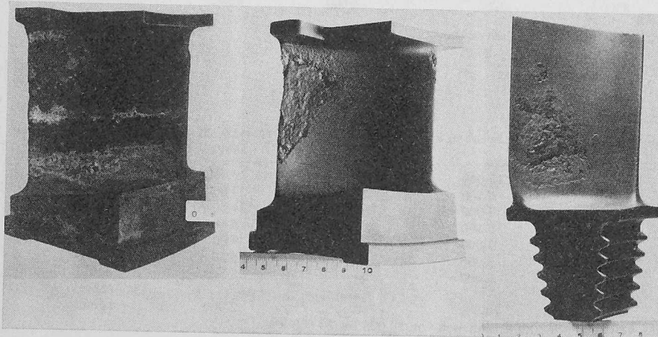
Bild 7. Leitschaufeln von Bild 6 nach Entfernung der Ablagerungen
