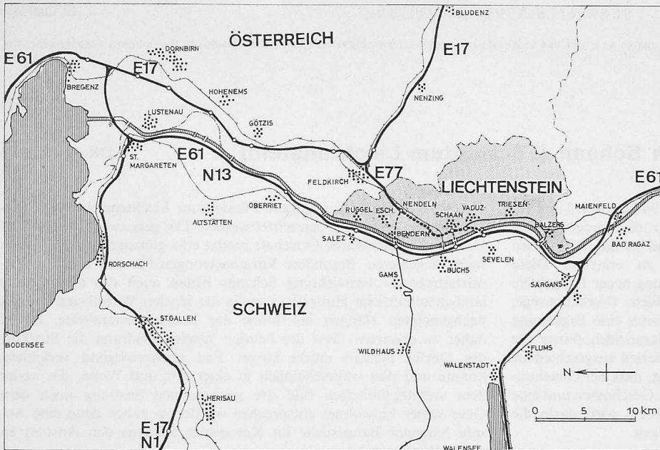
Bild 2. Projektierte und zum Teil ausgeführte Autobahnen und Hochleistungsstrassen in der Grenzregion Liechtenstein, Vorarlberg, Schweiz. Masstab 1:550 000 (ORL-Institut der ETH, Zürich)
