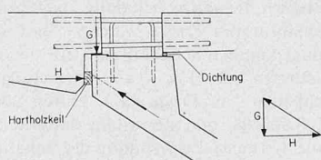
Bild 6. Anordnung der Keile zwischen Oberflansch und Fahrbahnplatte 1:25
