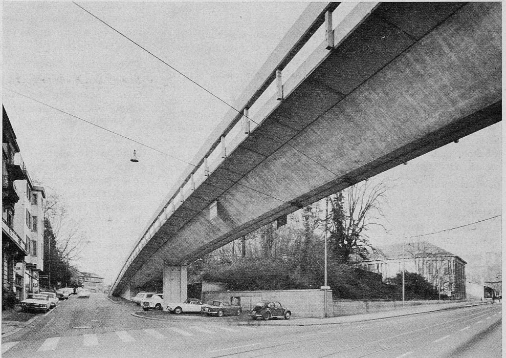
Bild 13. Fertige Brücke. Blick gegen Hirschengraben
