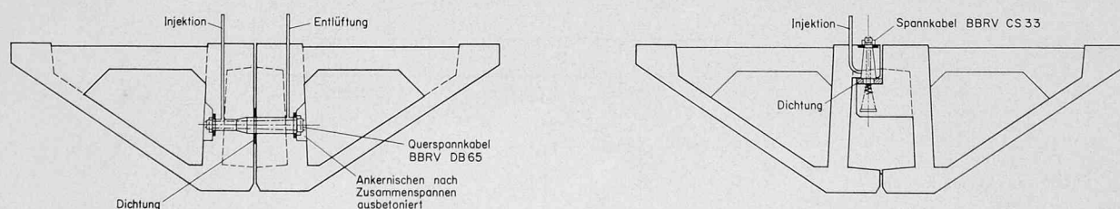
Bild 5. Verbindungsstellen zwischen den Trägerhälften. Links: vertikale Verbindung. Rechts: horizontale Verbindung. Masstab 1:50
