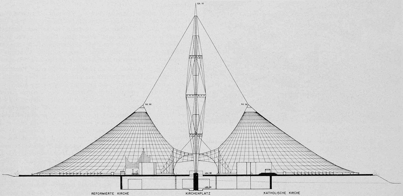
Längsschnitt 1:600
