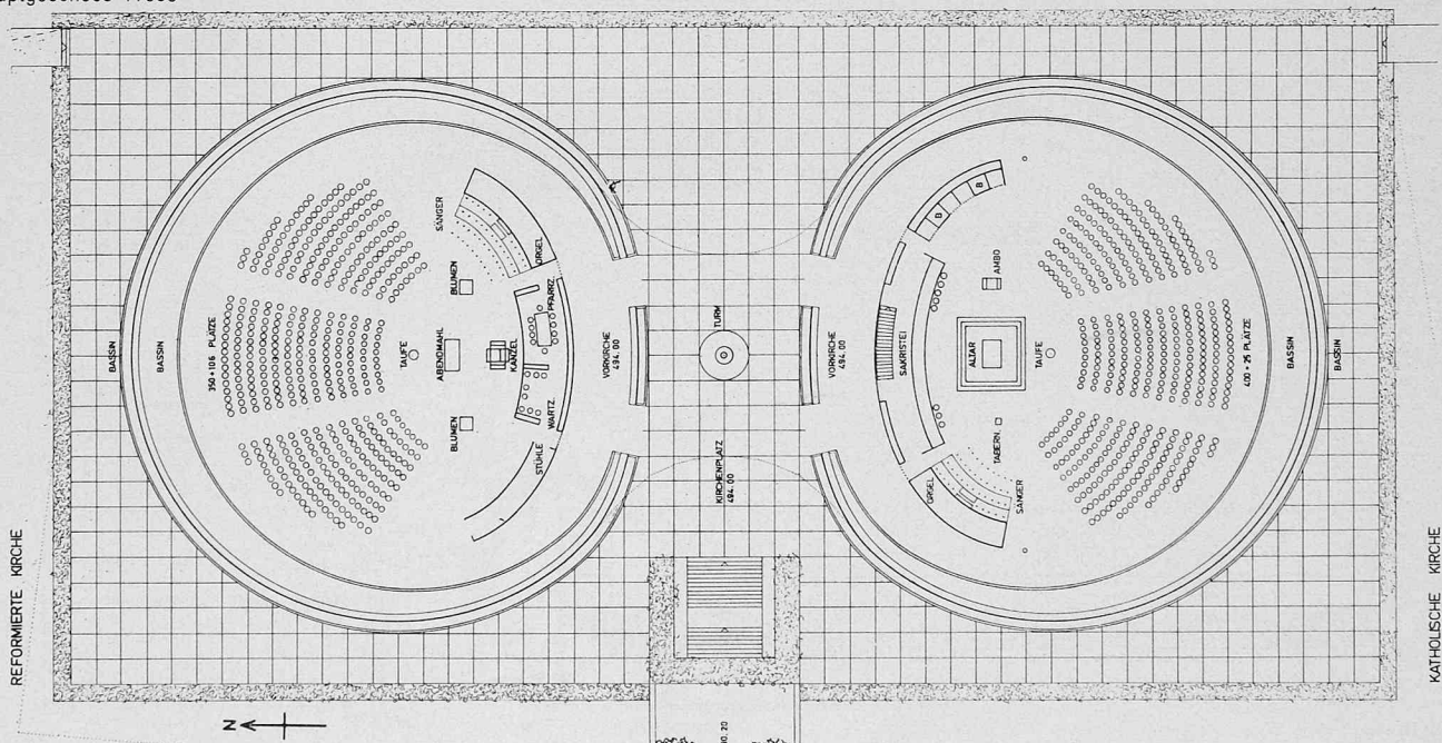
Hauptgeschoss 1:600
