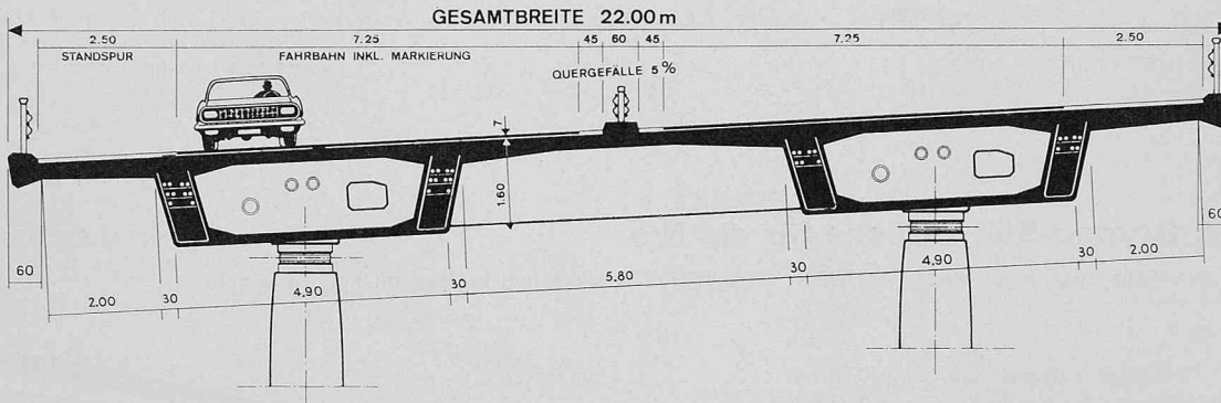
Bild 4. Normalquerschnitt 1:150
