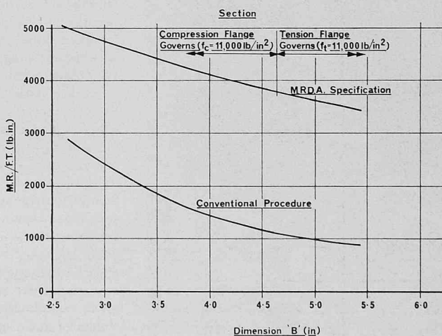
Bild 5 (rechts). Vergleich der Widerstandsmomente von Aluminiumblechtafeln bei konventioneller Berechnungsmethode und bei reduzierter Druckplattenbreite nach einer Formel auf Grund von Versuchswerten der «Metal Roof Deck Association» (Design and Technical Requirements for Light-Gauge Metal Roof Decks, October 1965):
