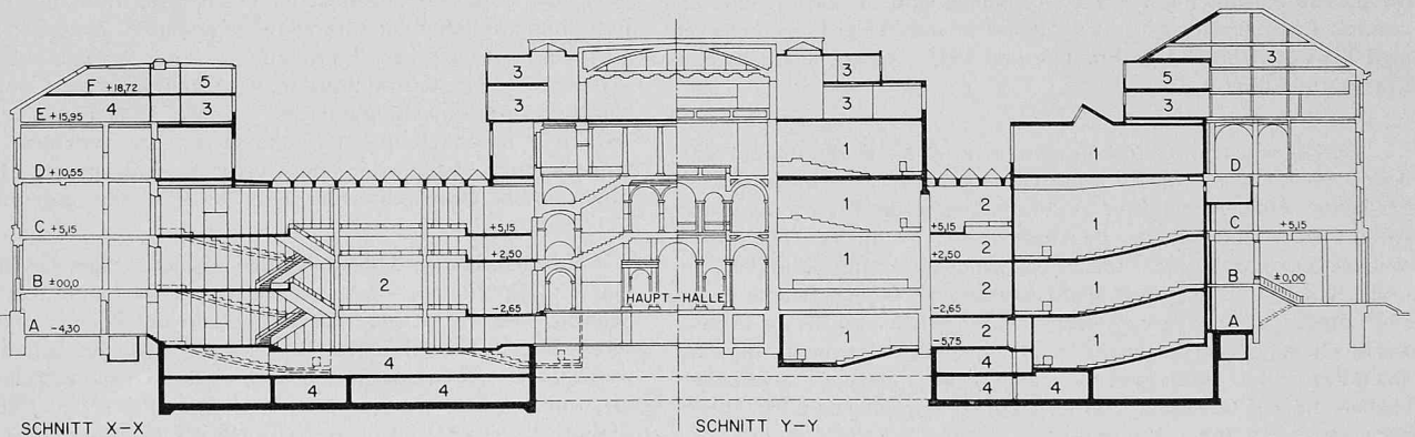
Bild 4. Kombiniertes Schnitt 1:800 durch den alten Bestand, die Hofeinfbauten und die übrigen Ausbauten im Hauptgebäude. Für die Schnittbezeichnung siehe Bild 3. Raumbezeichnungen: 1 Auditorien, 2 Foyers, 3 Bibliothek, 4 Bibliothek-Magazine, 5 Büroräume
