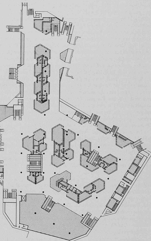
Bild 3. Erstes Tiefgeschoss, Masstab 1:1500. Gerasterte Flächen sind vorgesehen für Läden samt ihren Nebenräumen wie WC usw.
