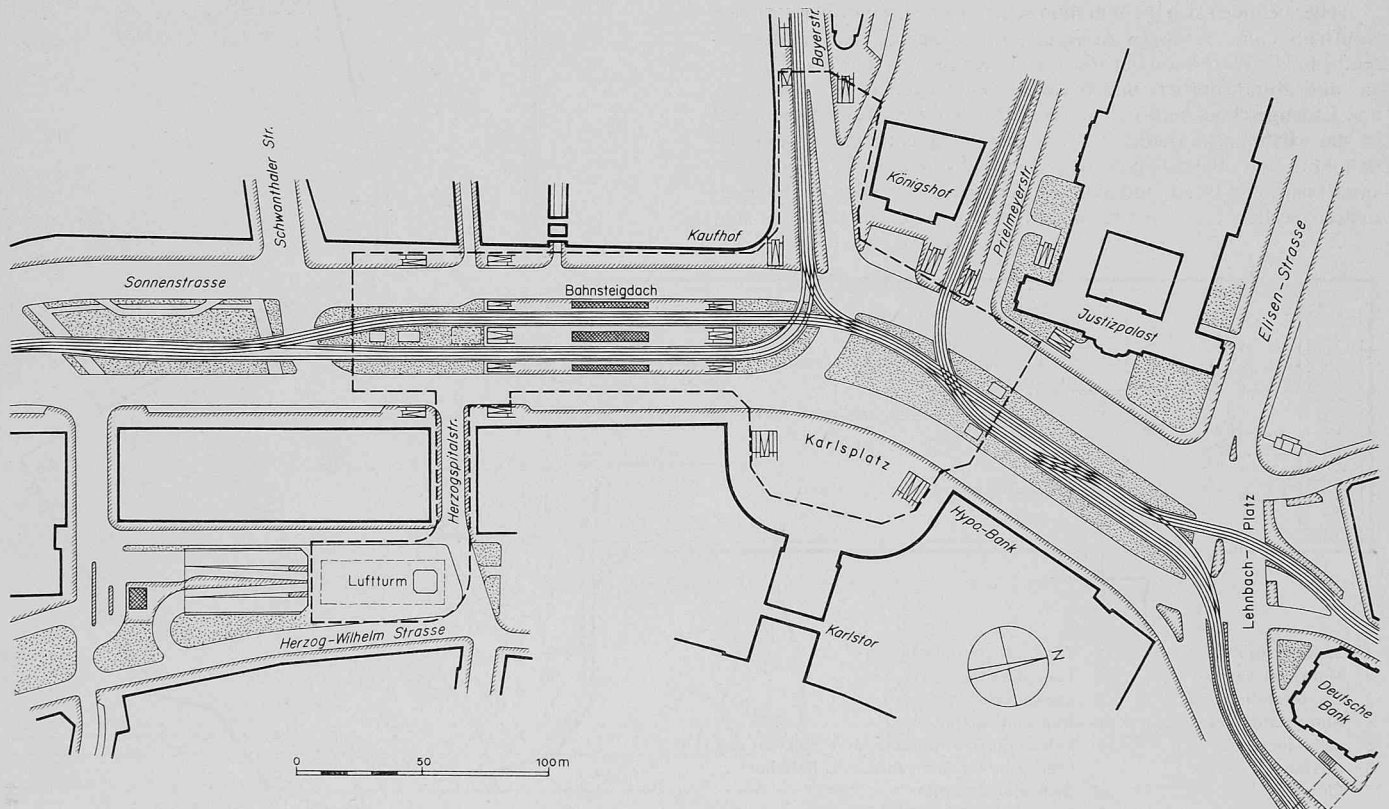
Bild 1. Der Stachus in München, Lageplan des Endausbaues, Masstab 1:3000. Gestrichelt ist der Verlauf der Schlitzwand eingetragen, deren Ausführungstapen in den Bildern 7 bis 11 durch fette Linien hervorgehoben sind
