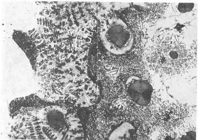
Bild 2. Gefüge der Schmelzlinie einer Lichtbogenschweissung von Gusseisen mit Kugelgraphit, ohne nachträgliche Wärmebehandlung
