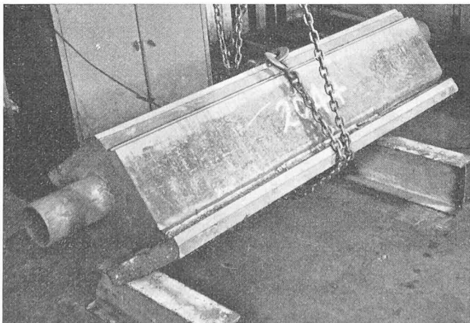
Bild 9. Maschinengestell aus Stahl mit aufgeschweisster Platte aus Gusseisen mit Kugelgraphit
