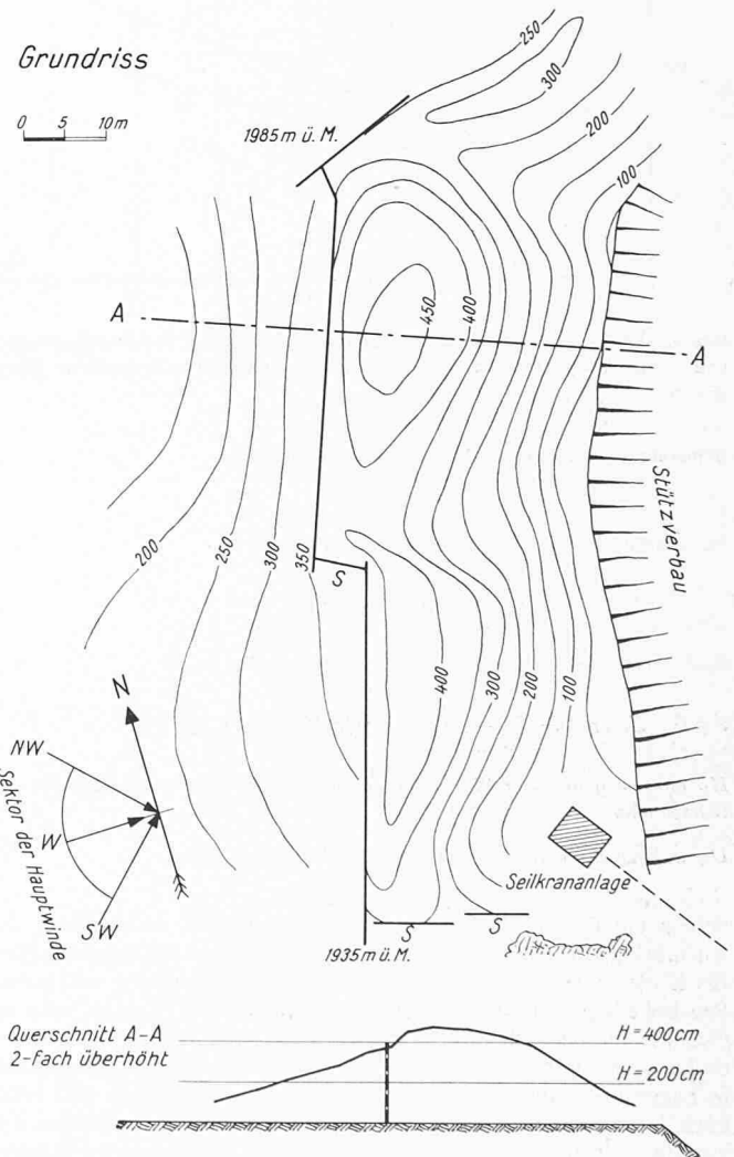
Bild 3. Triebsschneeeablagerungen am 14. April 1967 im Bereich der Triebsschneewände OeAM ( H = 400 cm) auf Fachswang, Lawinenverbauung Tanngrindel, Brienz. Die Triebsschneewände stehen ungefähr in der Hangfall-Linie und mehr oder weniger senkrecht zur Hauptwindrichtung. Die mittlere Hangneigung im Bereich der Triebsschneewände beträgt 29^\circ . S = Schneebrücken mit Füllungsgrad min. 65 %
