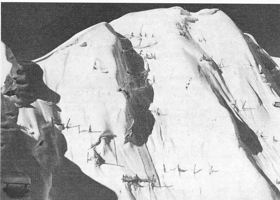
Bild 1. Stützverbauungen mit Schneenetzen im obersten Teil der Lawinanrissgebiete am Geissberg, 2375 m ü. M. (Gurtellen). Die steilsten Gipfelaufschwünge mit einer Hangneigung von über 45 ÷ 50° sind nicht verbaut und bilden das Anrissgebiet eines Schneebrettes mit seitlicher Ausbreitung in die verbaute Zonen. Unten links eine keilartig hinterfüllte Schneebrücke. Aufnahme 29. 1. 68 von W. Schwarz
