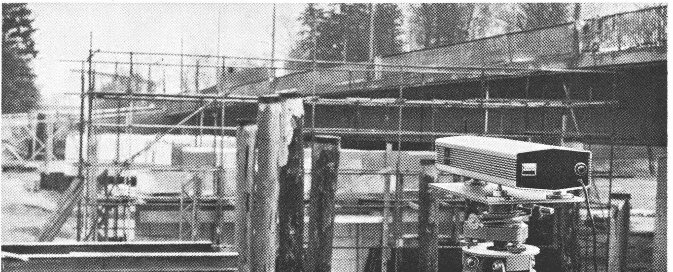
Siemens-Gas-Laser als optische Messhilfe auf einem Bauplatz
