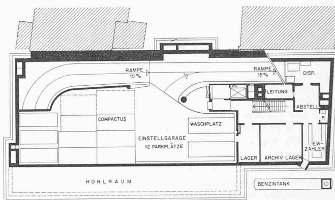
1. KELLERGESCHOSS
