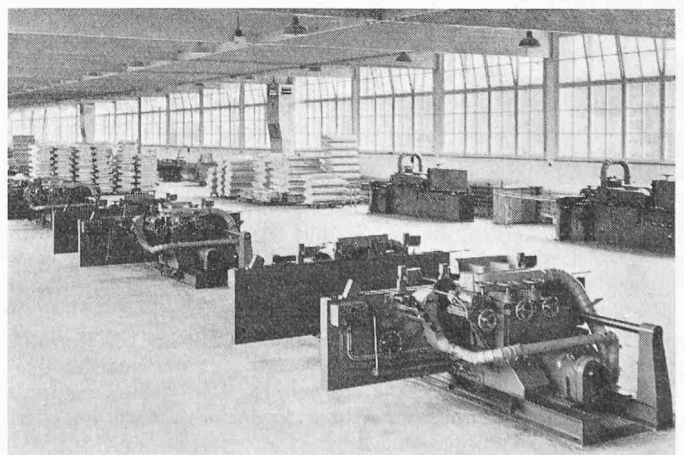
Fensterfabrik Kiefer in Rothrist. Im Vordergrund Zapfenschneidmaschinen-Gruppe
