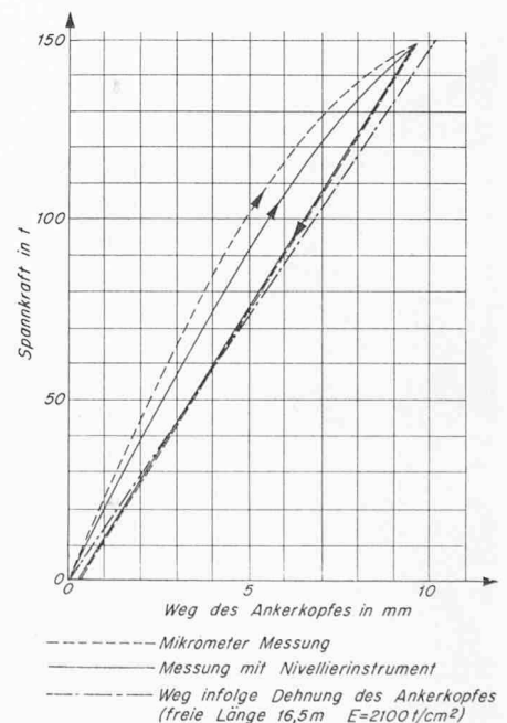
Bild 41. Zugversuch am Ankerpfahl Nr. 24, Spannungs-Dehnungs-Diagramme für den letzten Spannyklus auf 150 t
