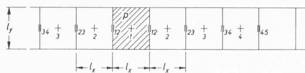
Bild 7. Bezeichnung der Biegemomente für den Hilfslastfall einer durchlaufenden Platte mit drei quadratischen Feldern und frei drehbar gelagerten Längsrändern
