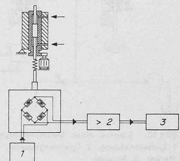
Bild 11. Druckmesser mit elektrischer Messeinheit
