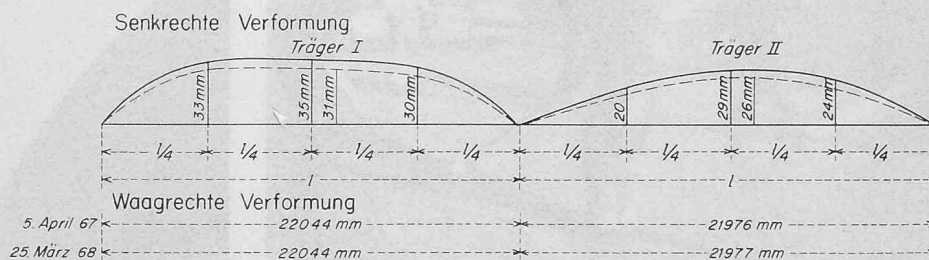
Bild 6. Verformung der Träger nach einem Jahr unter p = 0,3 \text{ t/m}^1 Nutzlast
