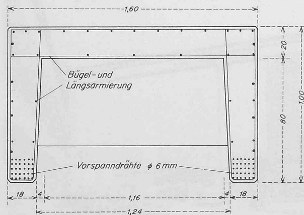
Bild 4. Trägerquerschnitt 1:25
