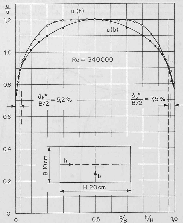
Bild 3. In Mittelschnitten des Rechteckrohres gemessene Geschwindigkeitsprofile mit Angabe der durch Integration bestimmten lokalen Grenzschicht-Verdrängungsdicken ( \delta^* ) bei Re = 340000
