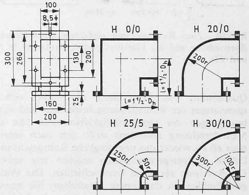
Bild 8b (links). Vier der Breitkant-Krümmer mit Angabe ihrer Kurzbezeichnungen und Konstruktionshinweisen
