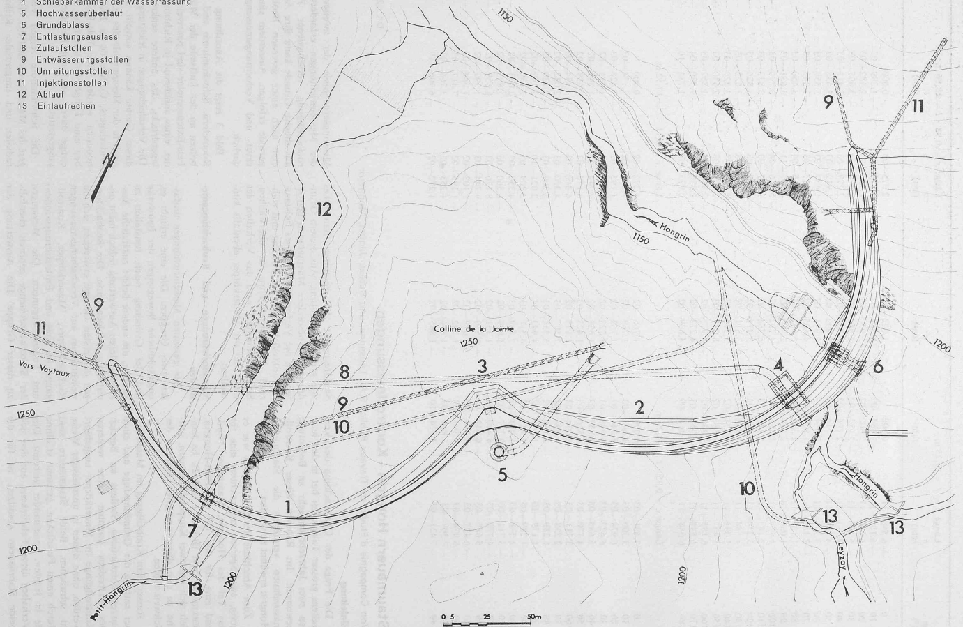
Bild 1. Grundriss
