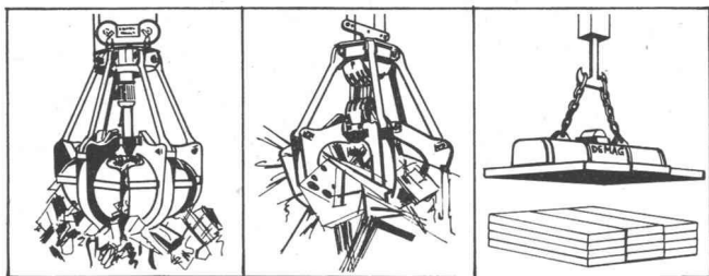
Polyp-Greifer für Kehricht Polyp-Greifer für Schrott Rechteck-Magnet
