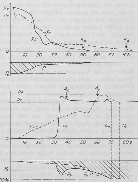
Bild 4 (rechts). Vorgänge beim Entleeren einer laufenden Pumpe
