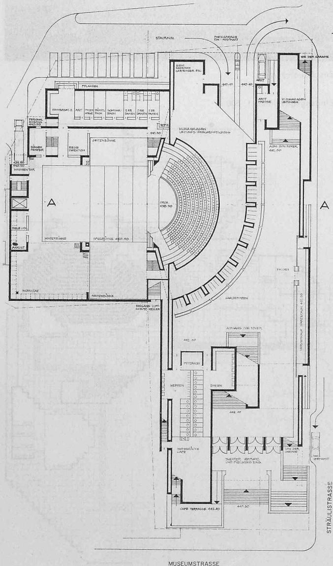
Erdgeschoss 1:800
