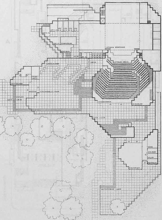
Eingangsgeschoss 1:800
