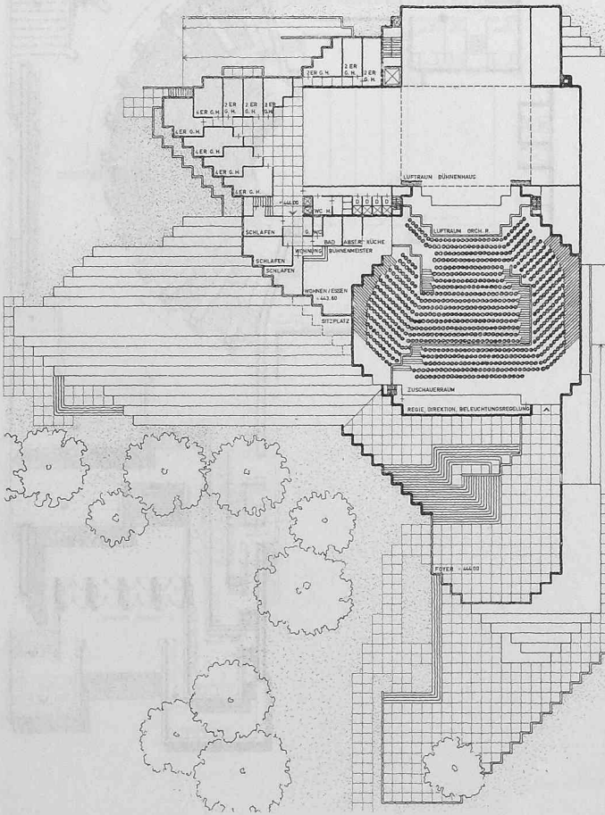
Obergeschoss 1:800
