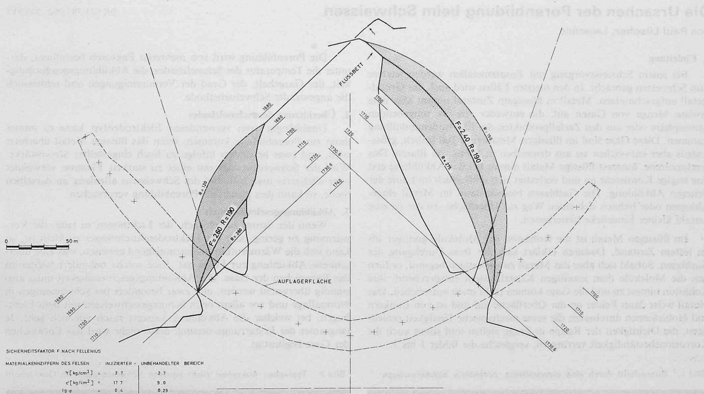
Bild 10. Stabilität der Widerlager für einen ausgewählten Schnitt
