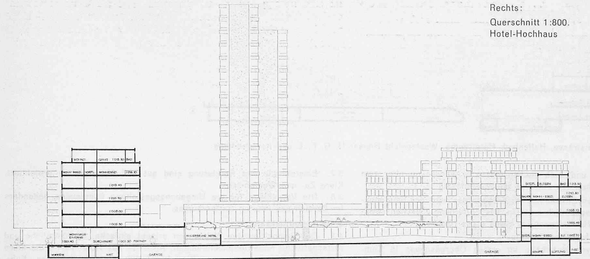
Längsschnitt 1:800. Durchfahrt, Haus A, Posthof, Garage, Haus F. Südansicht Hotel, Hallenbad, Personalhaus, Häuser G und H
