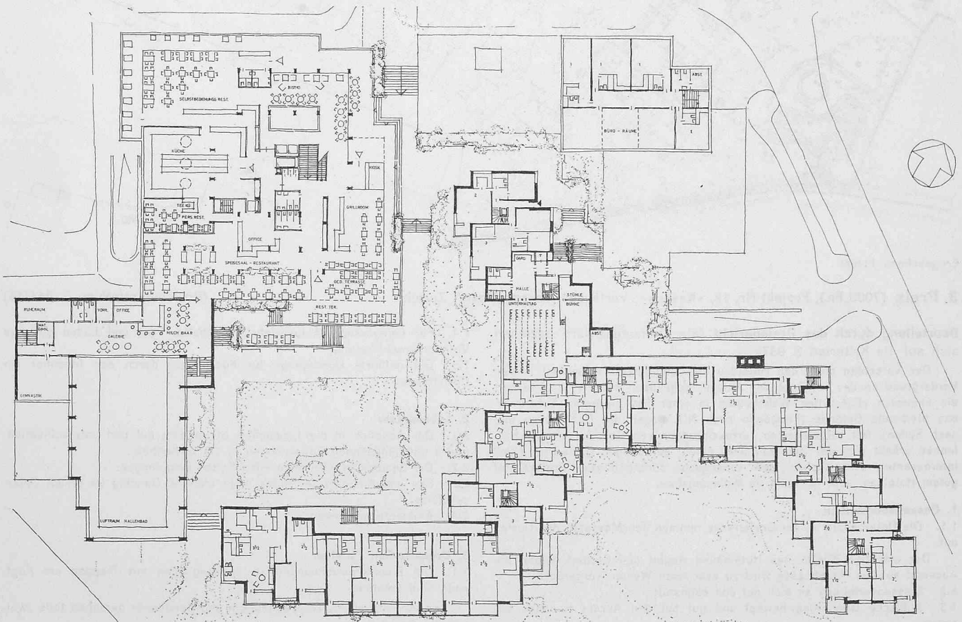
Erstes Obergeschoss 1:800
