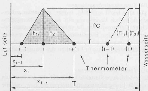
Bild 4. Verfahren zur Ermittlung der Einflüsse der einzelnen Thermometer auf einem Temperaturmesshorizont
