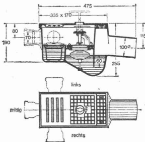
PRIMUS-Kellerablauf mit Rückstaudopperverschluss
