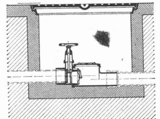
Rückstaudopperverschluss TRIPLEX für durch- gehende Leitungen
