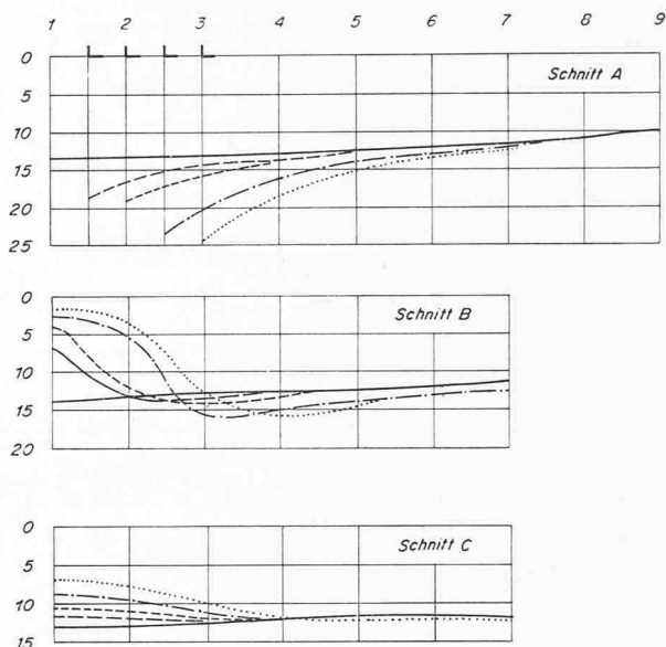
Bild 8. Gemessene Biegemomente [mt/m] der Versuchsserie III (Ausparung in Gurtstreifenmitte, «quer»)
