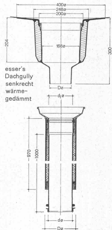
esser's zobelrohr doppelwandiger, wärmegeädmt Fallrohrstutzen für esser's Dachgullys, senkrecht
