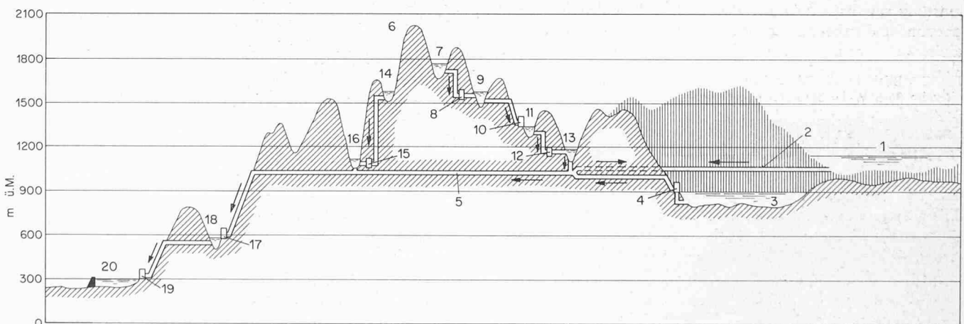
Bild 10. Schematisches Längsprofil des Murray-Systems. Die Kraftwerksanlagen bei Kosciusko, Windy Creek und Munyans wurden aus wirtschaftlichen Überlegungen weggelassen
