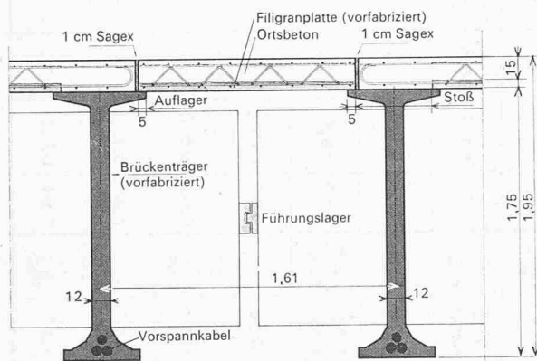
Tössüberdeckung in Winterthur. Querschnitt 1:45 durch das Tragwerk im Bereich der Dilatation zwischen zwei der je fünfstegigen Überbauelemente
