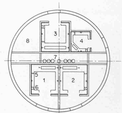
Bild 2. Grundriss des Fernsehturmes, schematisch 1 bis 4 Aufzüge 5 Initiatoren 6 Induktive Übertragung 7 Fernschleifungen 8 Raum für Treppen
