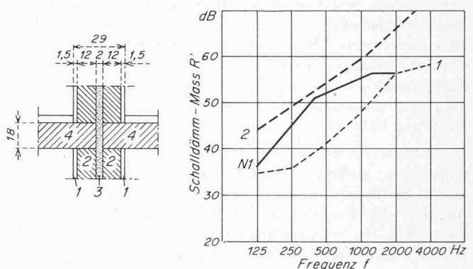
Bild 7. Luftschallisolierung einer Backstein-Doppelwand im Vergleich zu einer einfachen Backsteinwand von 12 cm
