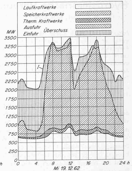
Bild 2. Vergleich der Mittwoch-Belastungen und der Erzeugungsarten im Sommer und im Winter des Jahres 1962
