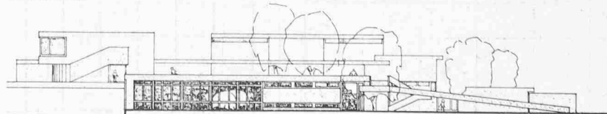
Nordfassade
