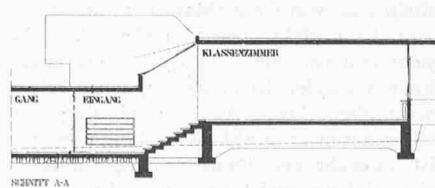
Schnitt A-A
