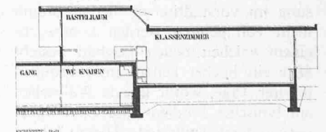
Schnitt B-B
