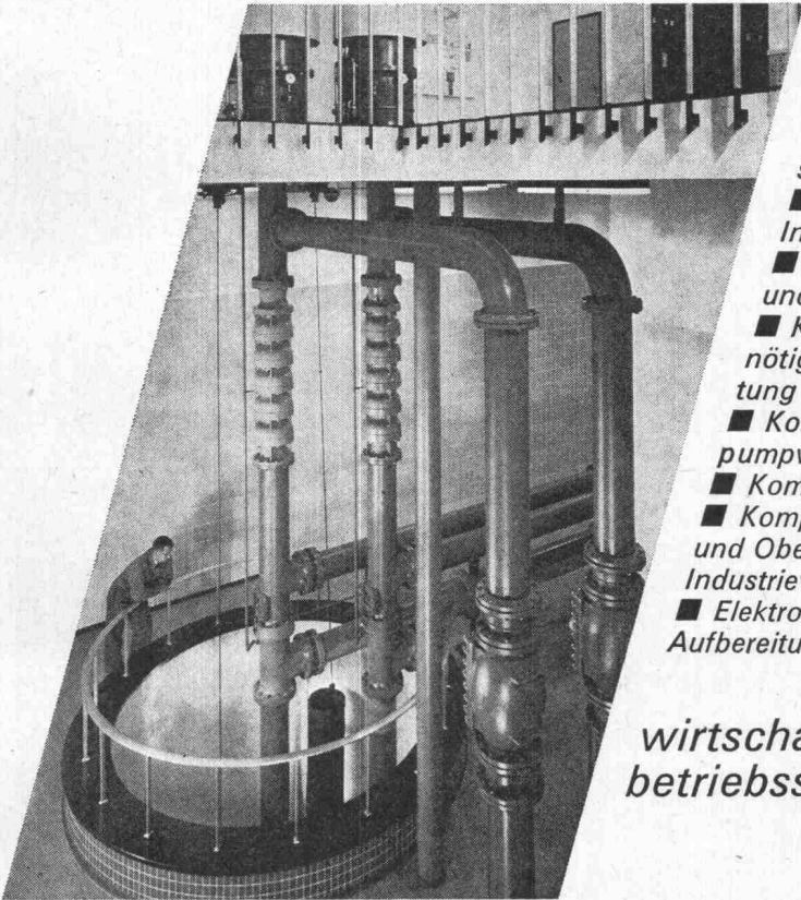
Grundwasserpumpwerk mit Sulzer-Bohrlochpumpen und einer Entkeimungsanlage durch Ozon
