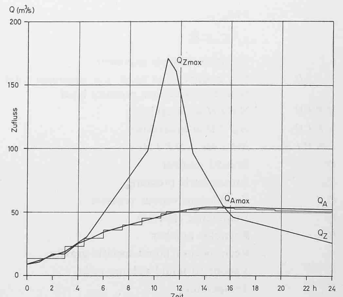
Bild 9. Zu- und Abflussganglinie des Hochwasserretentionsbeckens Orden
