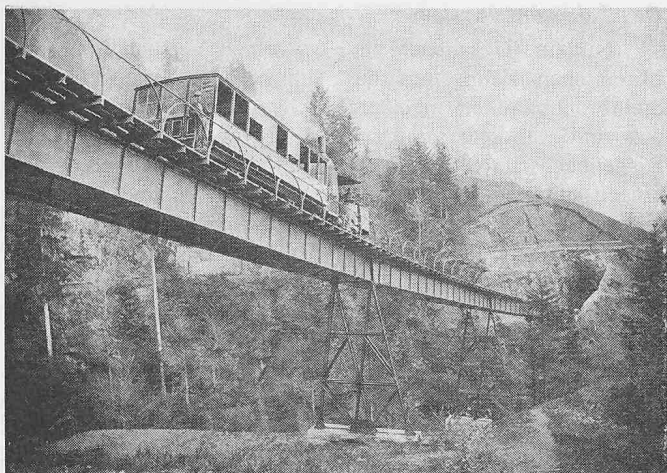
Bild 4. Schnurtobelbrücke im Originalzustand. Dampflokomotive mit stehendem Kessel
