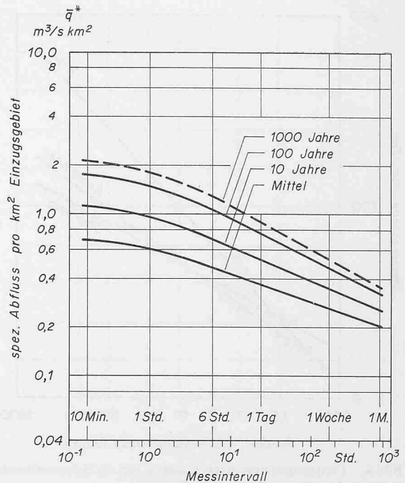
Bild 7. Spezifischer Abfluss \bar{q}^* ( \text{m}^3/\text{s} \cdot \text{km}^2 ) in Abhängigkeit von der Grösse des Messintervalles am Beispiel der Witenwasserreus bei Realp. Messperiode 1956/1970, Einzugsgebiet E = 30,7 \text{ km}^2
