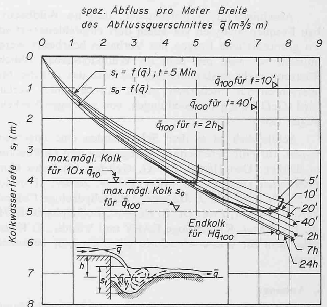
Bild 8. Kolkwasserstiefe eines hundertjährigen Hochwassers auf Grund der Frequenzanalyse nach Gumbel mit Abflussdaten von Bild 7, Breite des Abflussquerschnittes b = 7,0 m, Absturzhöhe h = 4,0 m, Korndurchmesser d_{95} = 1,00 m; \bar{q}_{10} = zehnjähriges Hochwasser, \bar{q}_{100} = hundertjähriges Hochwasser, H\bar{q}_{100} = hundertjährige Hochwasserspitze, s_t = Kolkwasserstiefe zur Zeit t
