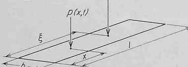
Bild 5. Berechnung der Lastschwankung für einen Streifen mit kontinuierlicher Druckverteilung
