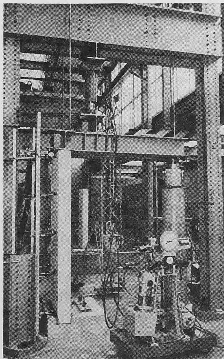
Bild 10. Versuchseinrichtung für Mauerwerkspeiler mit kombinierter Beanspruchung über Hochbaulager
