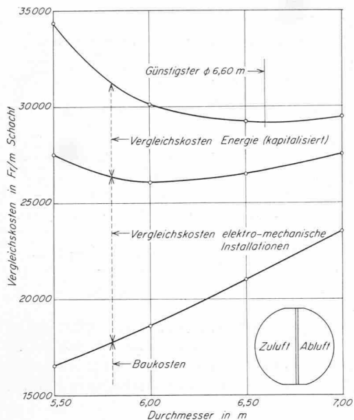
Bild 9. Ermittlung des wirtschaftlichsten Durchmessers für den Vertikalschacht Guspisbach. Die gesamte Luftmenge für Spitzenlastbetrieb (Zuluft und Abluft) beträgt 1148 m 3 /s. Darin ist die zusätzliche Reserve an Frischluft nicht enthalten. Es ergibt sich ein wirtschaftlicher Schachtdurchmesser von 6,6 m. Der Zuluftkanal bekommt eine Fläche von 18,0 m 2 , die günstigste Geschwindigkeit beträgt 31 m/s. Für den Abluftkanal errechnet sich die günstigste Fläche zu 14,2 m 2 , die günstigste Geschwindigkeit beträgt 39,5 m/s.
