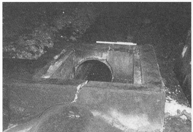
Bild 11. Zerstörung einer Tunnelsohle (Baujahr 1956) infolge Sohlenantrieb. Oberer Hauensteintunnel, Aufnahme Juli 1972
