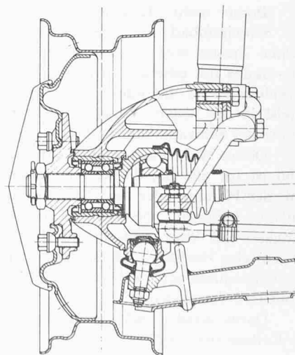
Lagereinheit in Form zweireihiger Schrägkugellager als Vorderadler in einem Personenwagen (Werkbild SKF)
