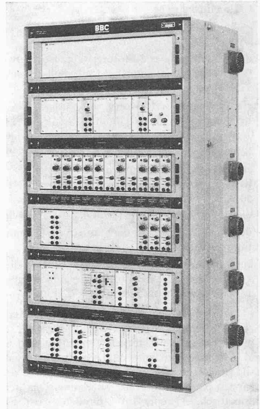
Bild 41. Elektronikschrank BBC
