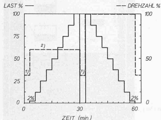
Bild 22. US-Federal-Dieselzyklus. 1 Leerlauf; 2 Entweder 60 % der Nennzahl oder Drehzahl des maximalen Drehmoments, je nach dem, welche höher liegt
