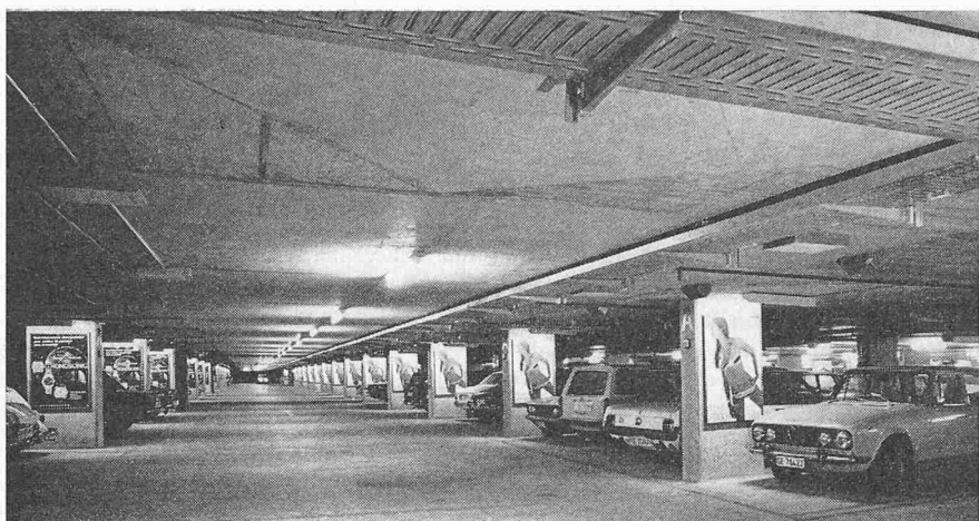
Gesamtansicht einer Etage der fertigen Unterwasser-Parkgarage in Genf
