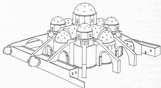
Schaubild 1:600 der Klosterkirche von Perissa. Eine Hauptkuppel mit Tambour von 8,25 m Durchmesser schwebt über der Vierung der tonnengewölbten Kreuzarme, die in Halbkreis-Apsiden endigen. Unter dem Tonnenkämpfer öffnen sich die Arkaden zu den Neben-Kuppelräumen, die ihrerseits an den beiden Aussenseiten nochmals durch Segmentapsiden ausgeweitet werden. Dieser grossartige (heute etwa 200 Jahre alte) Zentralbau wird von weitausholenden Strebebögen abgestützt, die in der Höhe der Tonnenkämpfer angreifen ... Möglicherweise hatte der Erbauer der Perissa-Kirche französisch-geothische Kathedralen auf Zypern gesehen; dann hat er aber mit souveränem Verständnis frei über diese Anregung verfügt, so dass etwas durchaus Eigenes daraus geworden ist – ein Unikum in der byzantinischen Architektur ... (nach dem Artikeltext ausgezogen)
