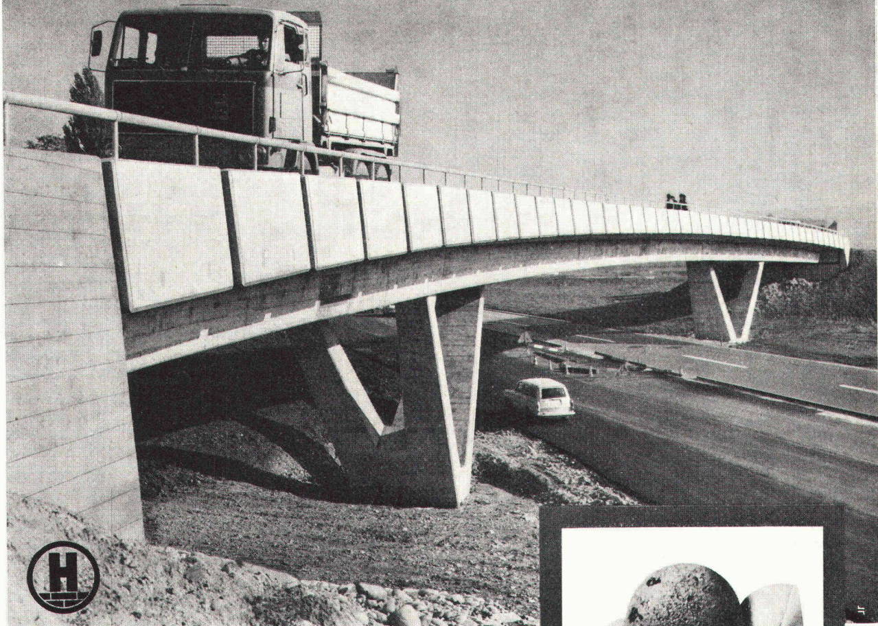
Brücke aus Leca h 2 d e -Beton beim N 4-Anschluss (Mutzentäli), Schaffhausen Bauherr: Tiefbauamt des Kantons Schaffhausen Statik: Wehrli & Weimer, dipl. Bauing. ETH/SIA, Zürich Bauausführung: B. Ehrat-Osswald, Baugeschäft, Neuhausen am Rheinfall
