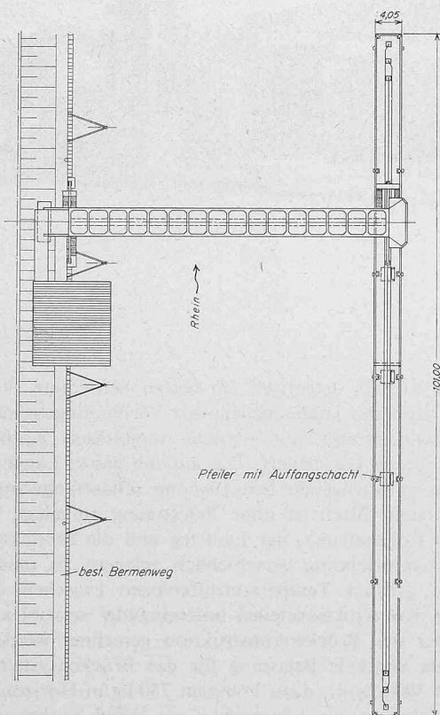
Bild 3. Grundriss 1:1000
