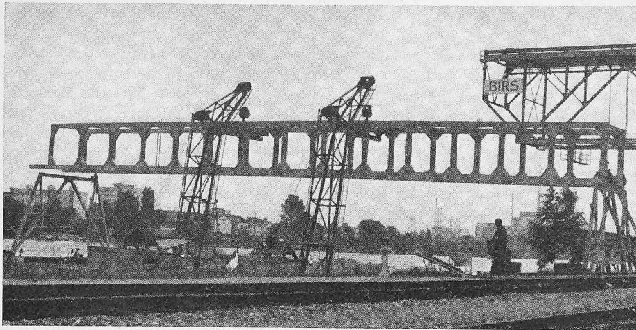
Bild 1. Mit einem präzisen Einschwimmmanöver wurde es möglich, die Brücke in zwei Stunden auf die vorbereiteten Auflagerjoche zu montieren. Schutzwanne, Rohrleitungen, Laufsteg, Aufstiegstreppen, die Kabine für den Leitstand und die Elektroinstallationen konnten anschliessend von den jeweiligen Unternehmern gefahrlos und ohne Beeinträchtigung des Schiffs- und Verladebetriebes ausgeführt werden
