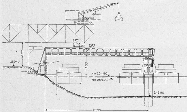
Bild 2. Ansicht von Oberstrom 1:1000
